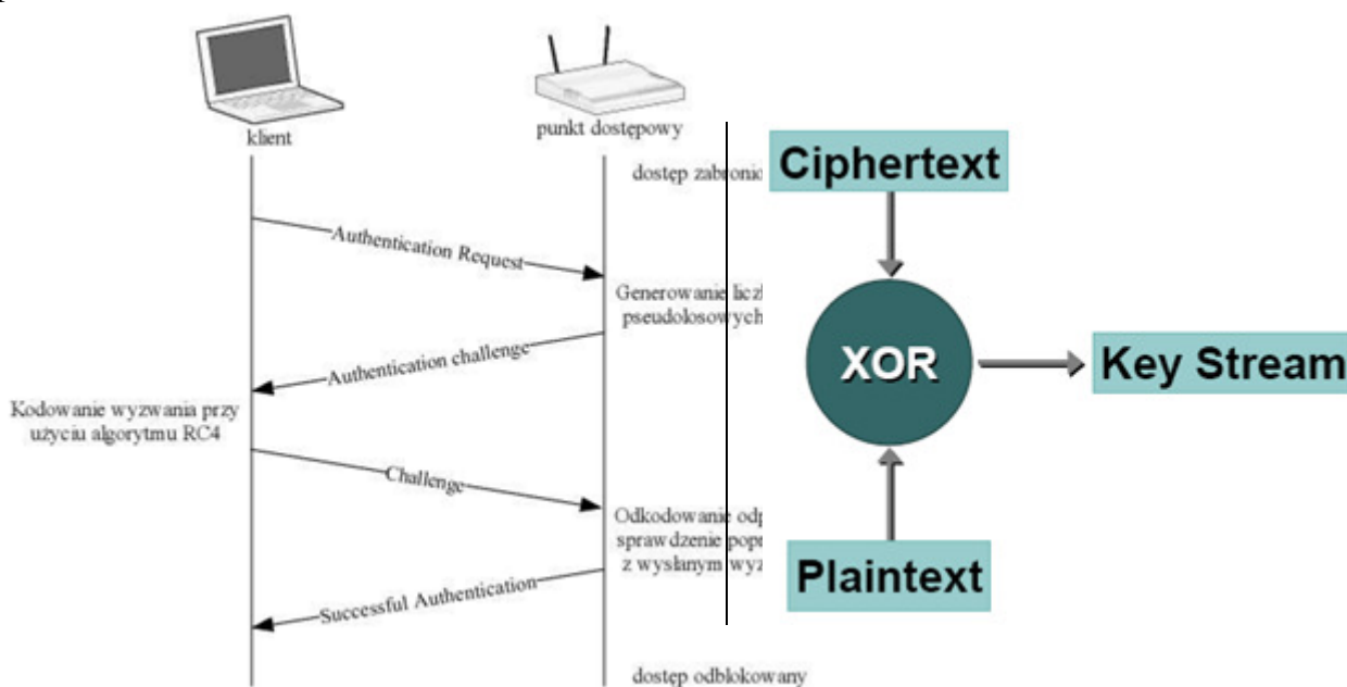
Rys. Uwierzytelnianie shared-key i metoda uzyskania ciągu szyfrującego.
