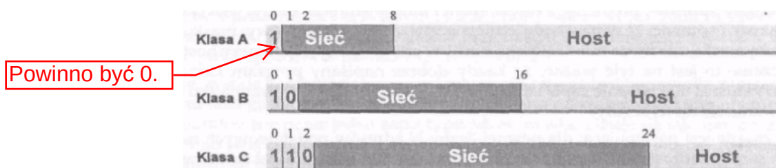
Rysunek 1 -4: Klasa adresu jest zakodowana w pierwszych kilku bitach
